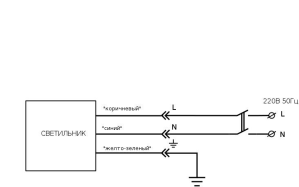
Рисунок 1. Электрическая схема подключения.
