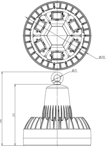
Рисунок 2. Габаритный чертеж
